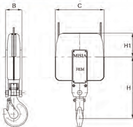
S2 (2/1) GANCI NORMA DIN 15401 - HOOKS STANDARD DIN 15401
