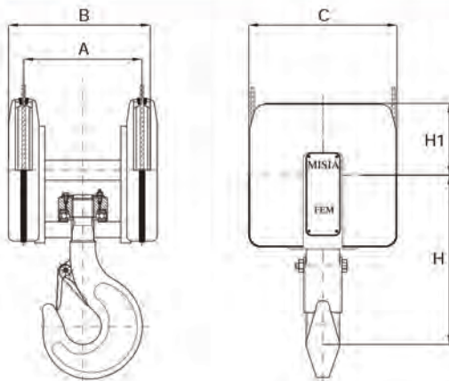
S4 (4/1) GANCI NORMA DIN 15401 - HOOKS STANDARD DIN 15401
